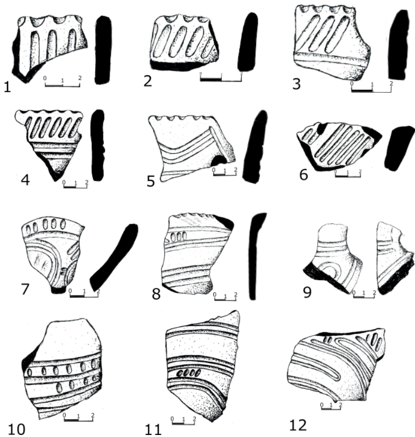
Рис. 1. Керамічна колекція з поселення Тополі: варіації із заглибленим орнаментом; 7-8 – композиція доповнена канелюрами
