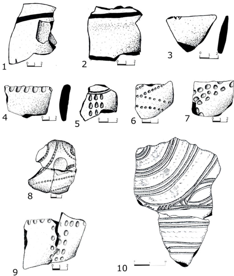
Рис. 2. Керамічна колекція з поселення Тополі: 1-3 фрагменти кераміки із розписом; 6-7 – фрагменти кераміки з круглим штампом; 10 – фрагмент грушоподібної посудини
